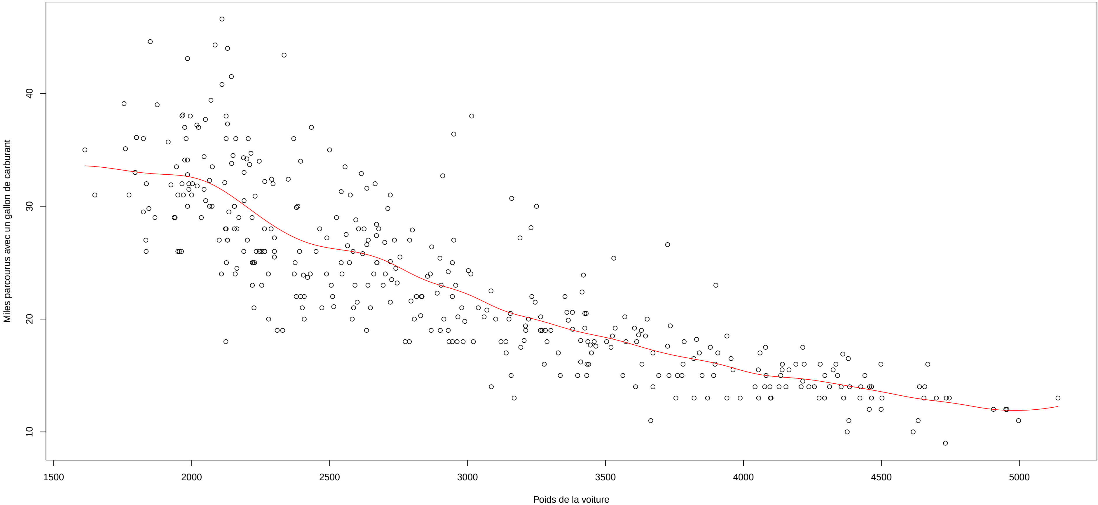
Estimateur de Nadaraya Watson avec h=h.min
